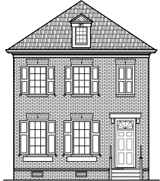
B2 OPTIONAL ELEVATION
