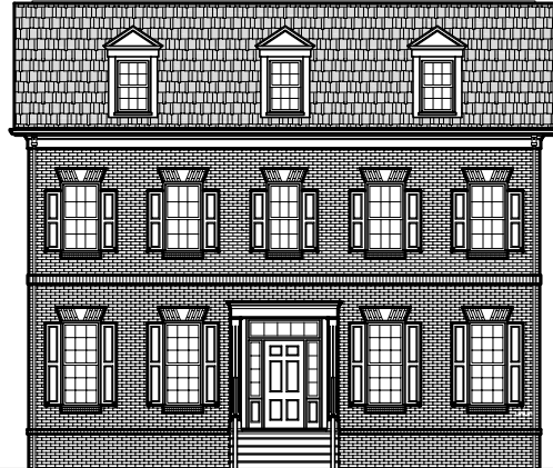
B2 - OPTIONAL ELEVATION
