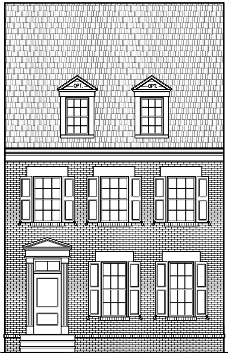
B3 ELEVATION
