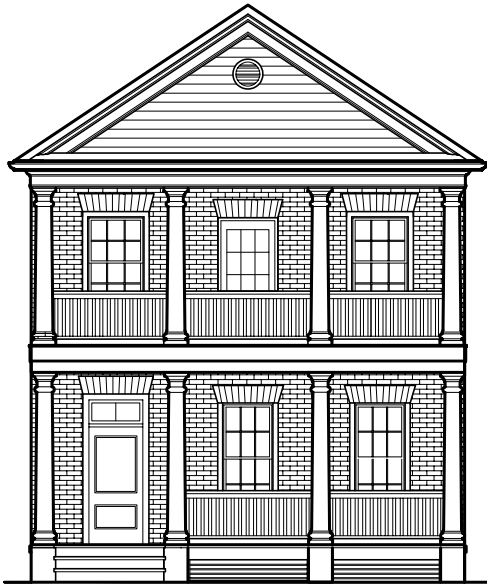
B4 OPTIONAL ELEVATION
