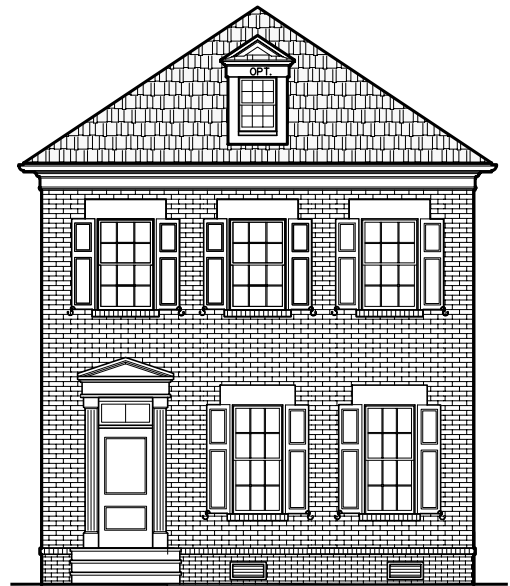
B3 OPTIONAL ELEVATION
